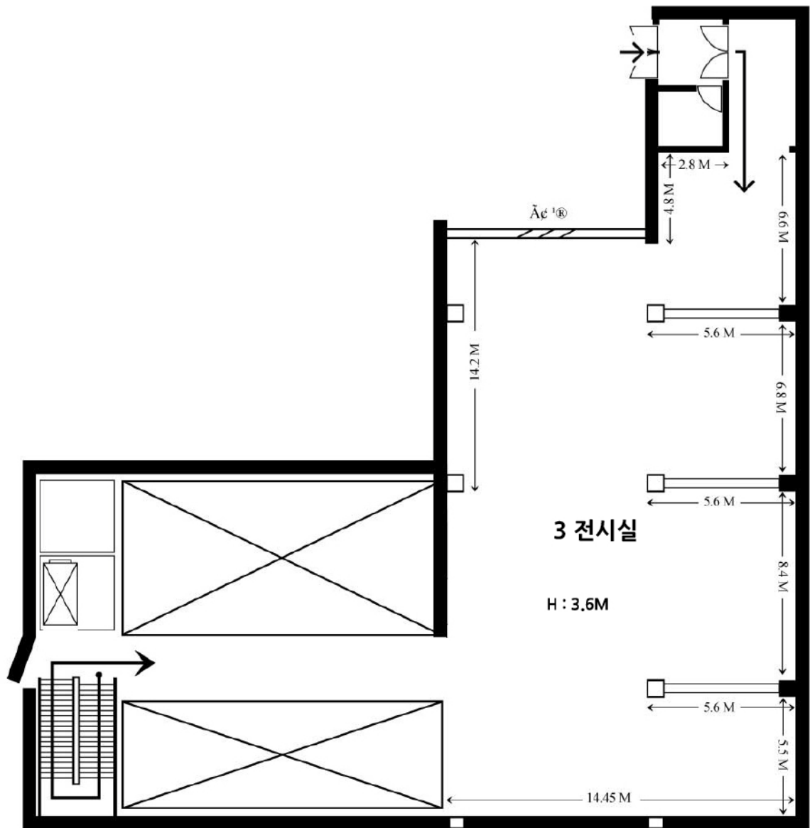
한국소리문화의전당 전시장 3F 평면도
