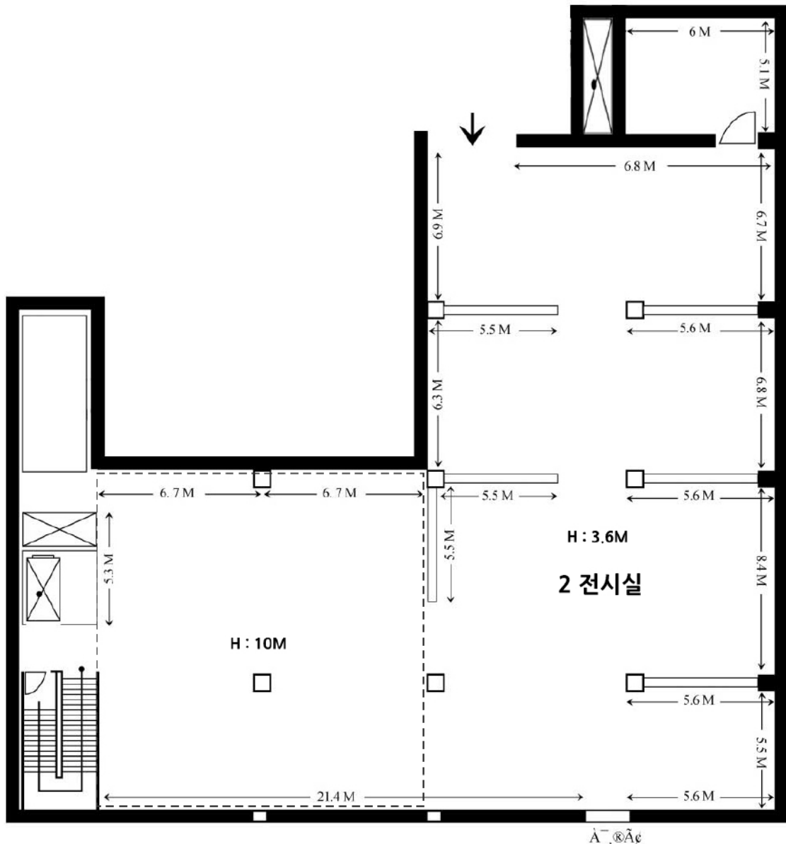
한국소리문화의전당 전시장 2F 평면도
